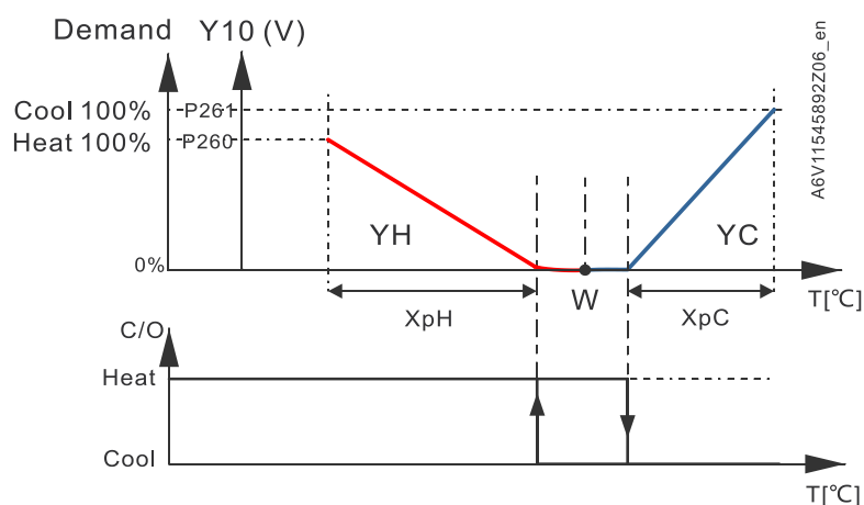
Hydraulické a řídicí schéma regulační sekvence 6-cestného PICV
