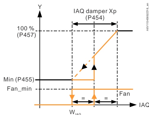
Mrtvé pásmo (P458 = ON)
