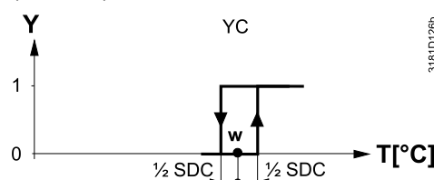
Režim chlazení s ruční předvolbou (P001=3)
