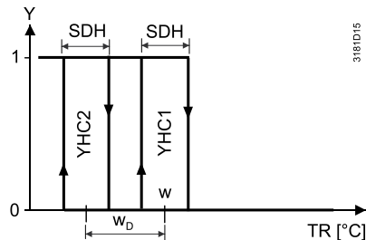
Režim vytápění (P001 = 0)
