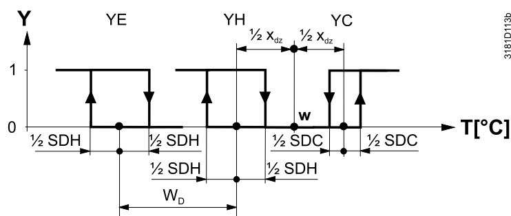
Vytápění a chlazení (P001 = 4)
