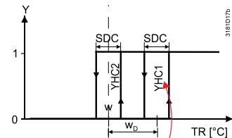
Přepínání (P001 = 2 nebo P001 = 3, P254 = 1) (funkce změny pořadí výstupů)
