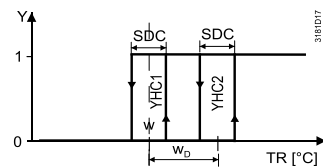
Přepínání (P001 = 2 nebo P001 = 3, P254 = 0)
